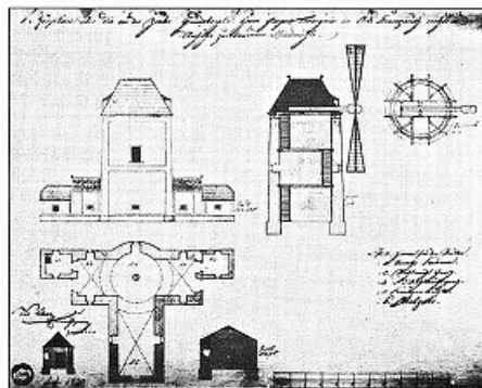
Plán větrného mlýna ve Štrampouchu zhotovený pro markýze de Trazegnies roku 1820
